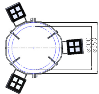
DIMENSIONES
