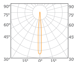
SUPER CONCENTRADA 10°
