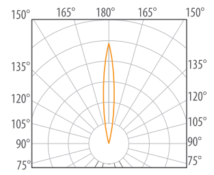
CONCENTRADA 14°
