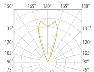
DIFUSA 40°
