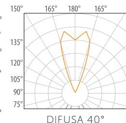
PARA INSTALACIÓN EMPOTRADO EN MURO
